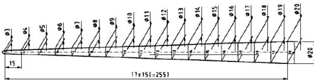
Рисунок 1 - Приспособление для измерения способности к вязке узлов К
