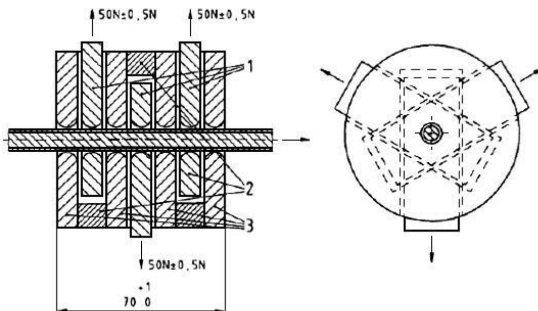
1 - движущиеся пластины; 2 - пространство; 3 - закрепленные пластины
