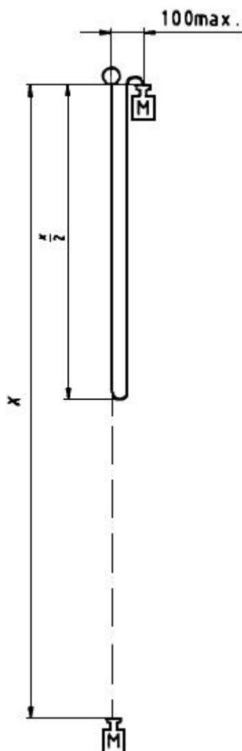
Рисунок 9 - Определение динамической прочности (см. 5.9.5)
